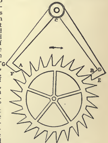
FIG. 9.—Dead Escapement.
